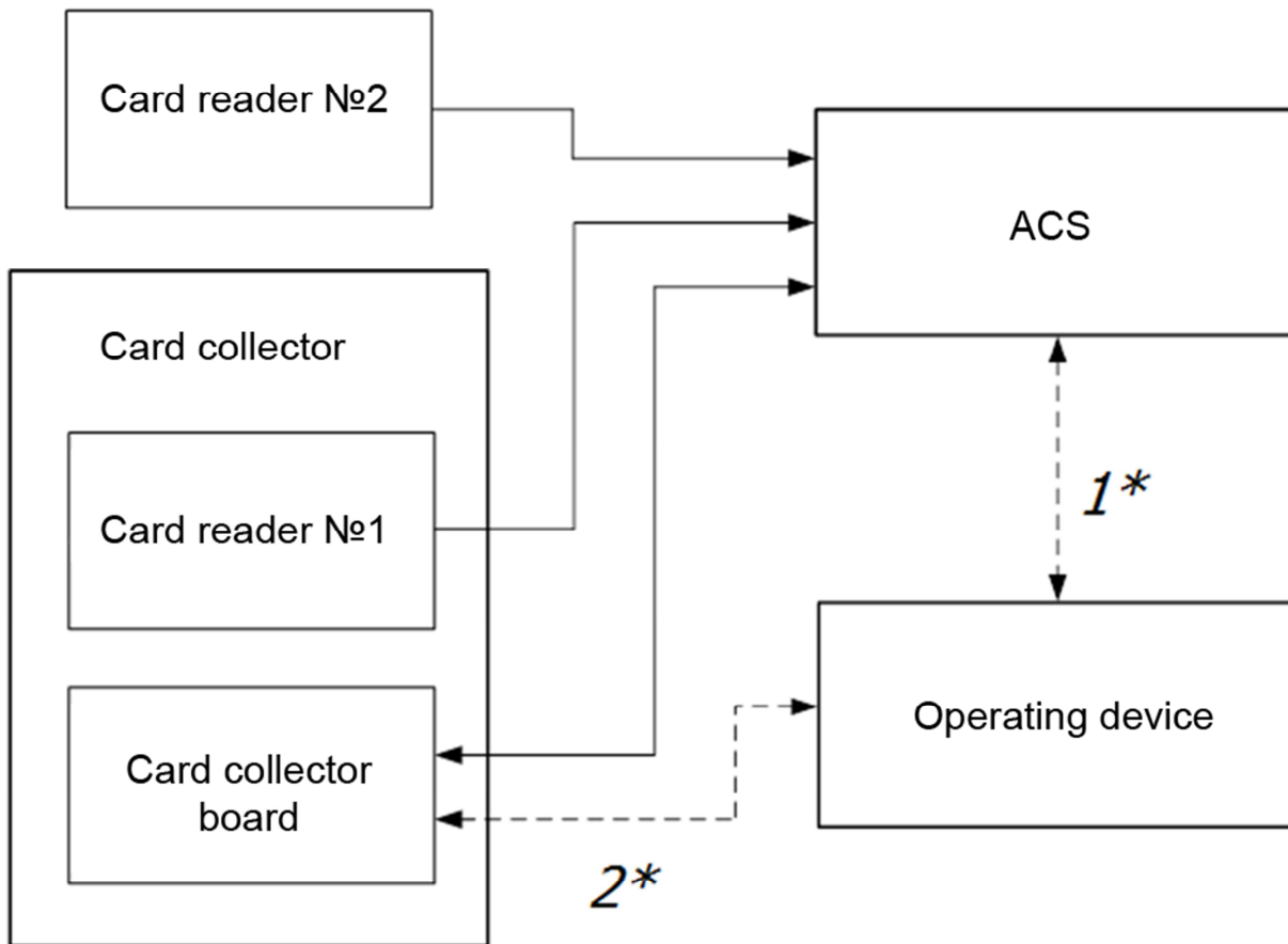
Fig. 20. Block diagram №1
